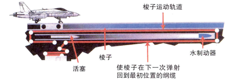
/ 航母弹射器构造示意图。
