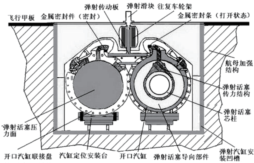
/ 美国航母上使用的弹射器开口汽缸组件截面示意图。
